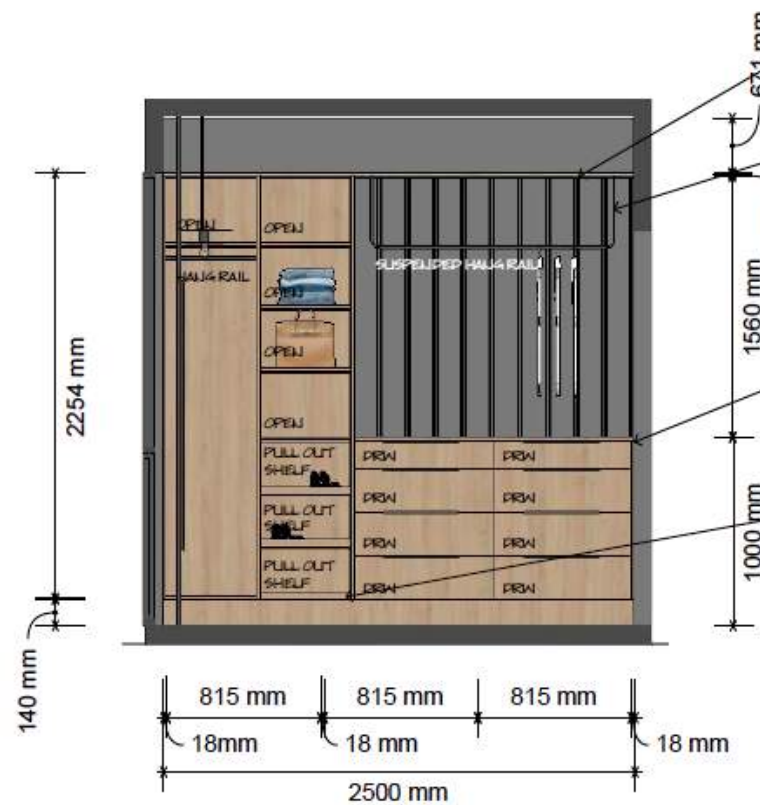
L WIR SECTION 1:40 @ A3
