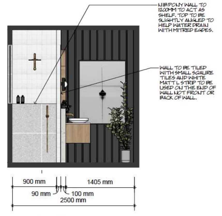
SECTION D 1:40 @ A3
