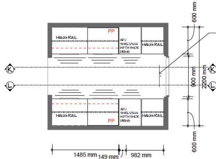
WIR FLOOR PLAN 1:40 @ A3
