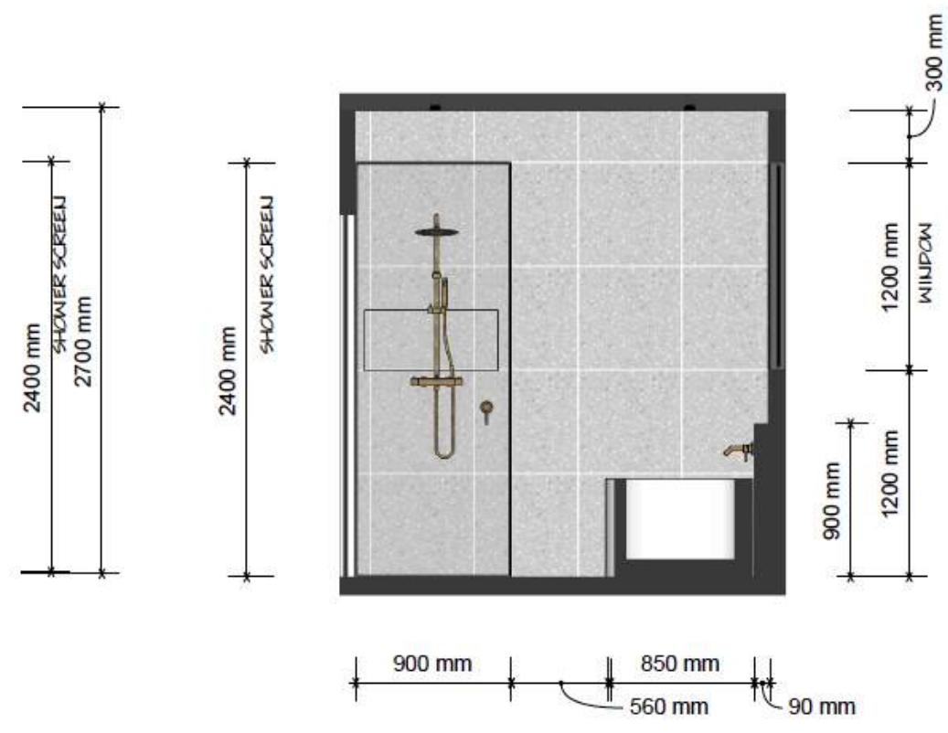
G SECTION 1:40 @ A3
