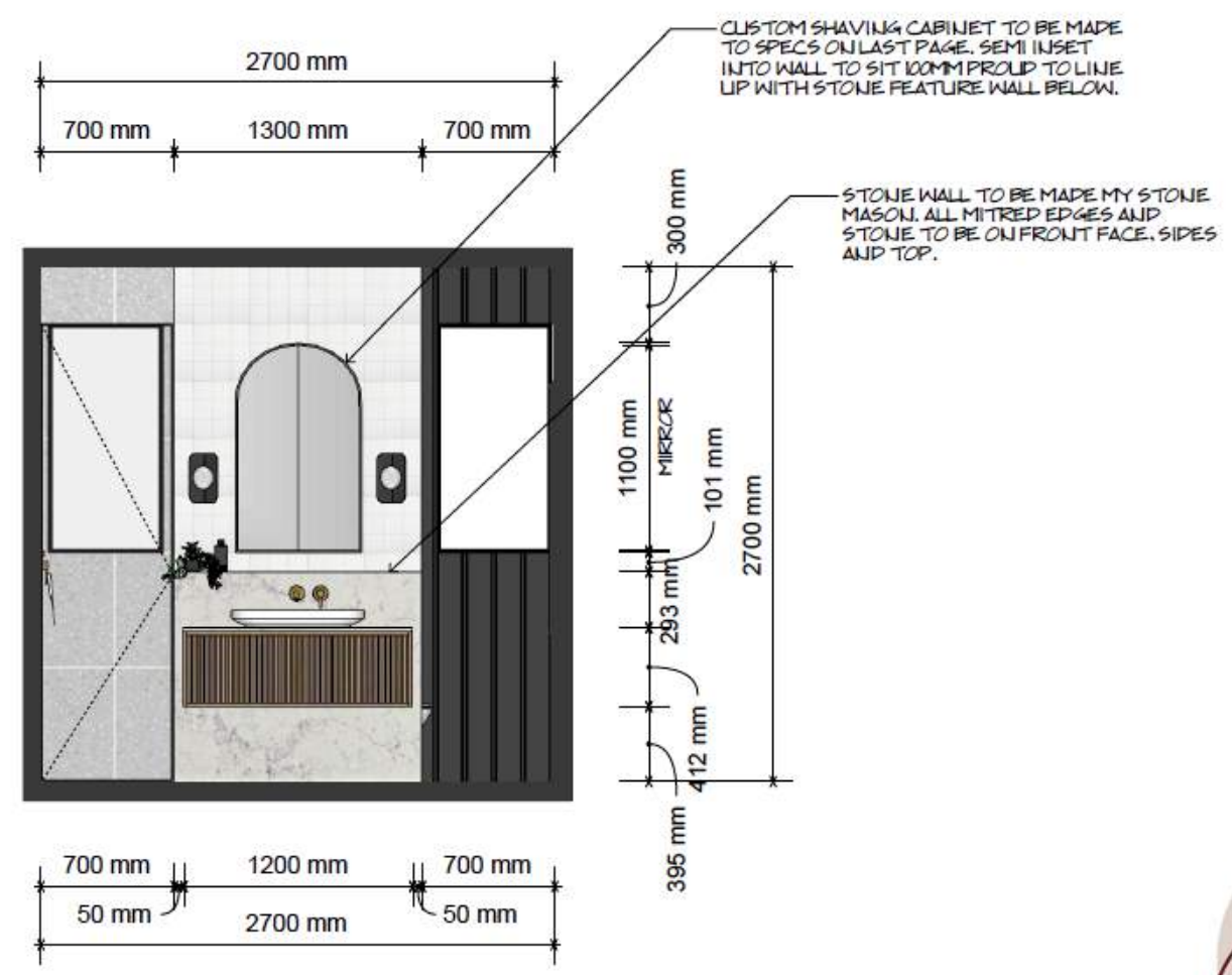
SECTION A 1:40 @ A3
